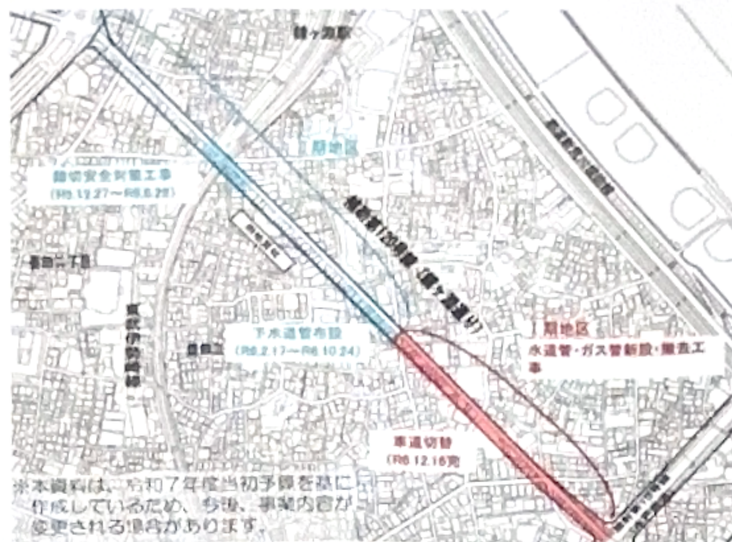
工事実施予定箇所図(一部抜粋)
